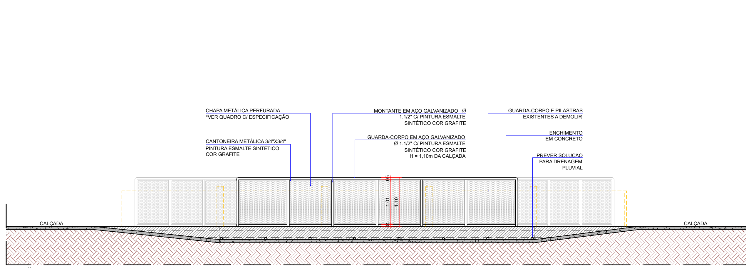
SEÇÃO AA - PONTE NA RUA SERRA FORMOSA ESCALA 1:50
