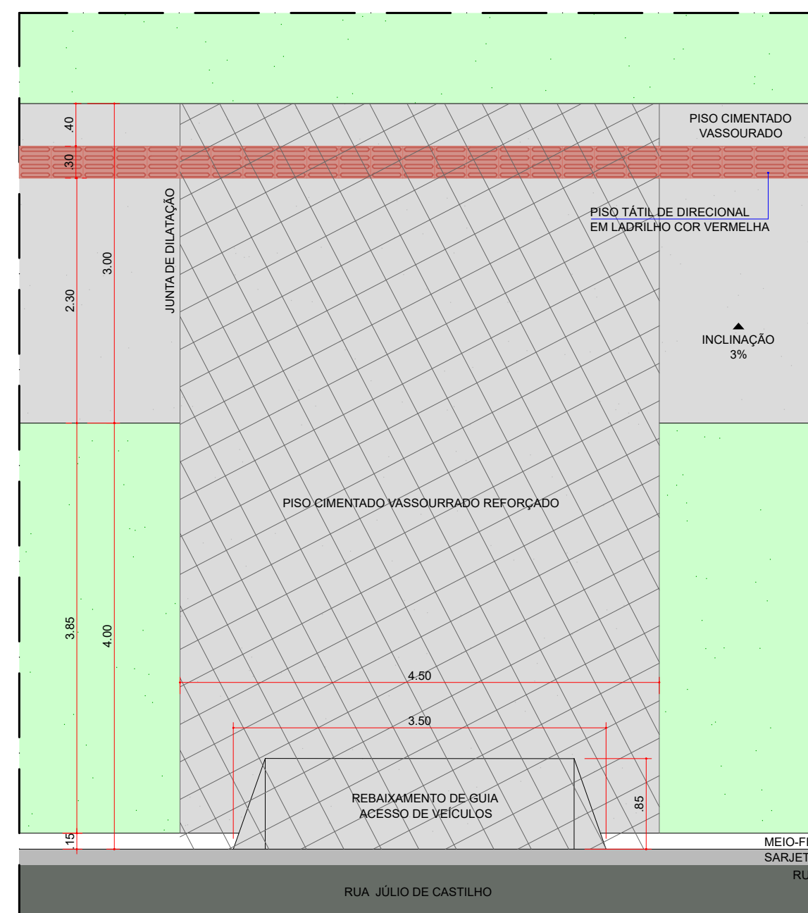
DETALHE 3 - REBAIXO DE GUIA ESCALA 1:50
