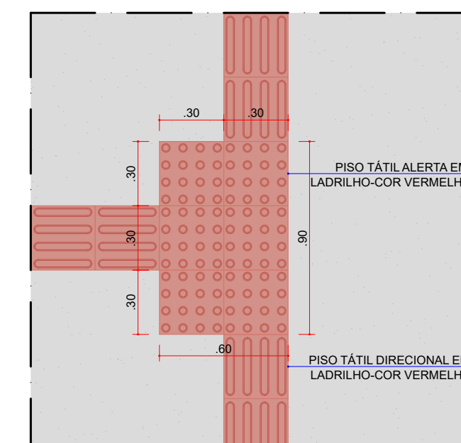
DETALHE 9 - PISO TÁTIL 90° ESCALA 1:25
