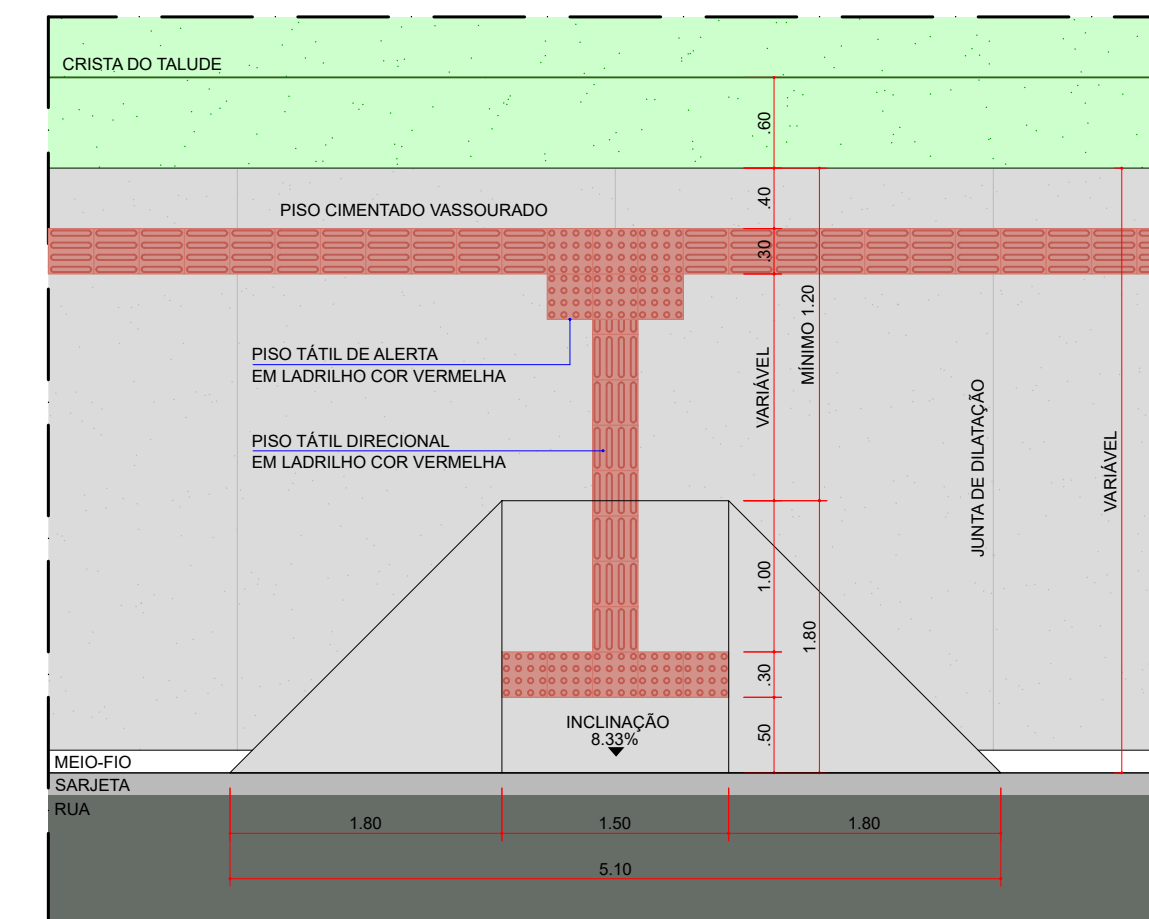
DETALHE 5 - RB1 (REBAIXO DE GUIA P.N.E. TIPO 1) ESCALA 1:50
