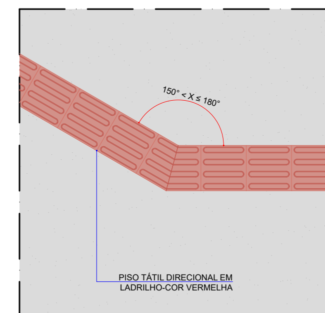
DETALHE 8 - PISO TÁTIL DIRECIONAL ESCALA 1:25
