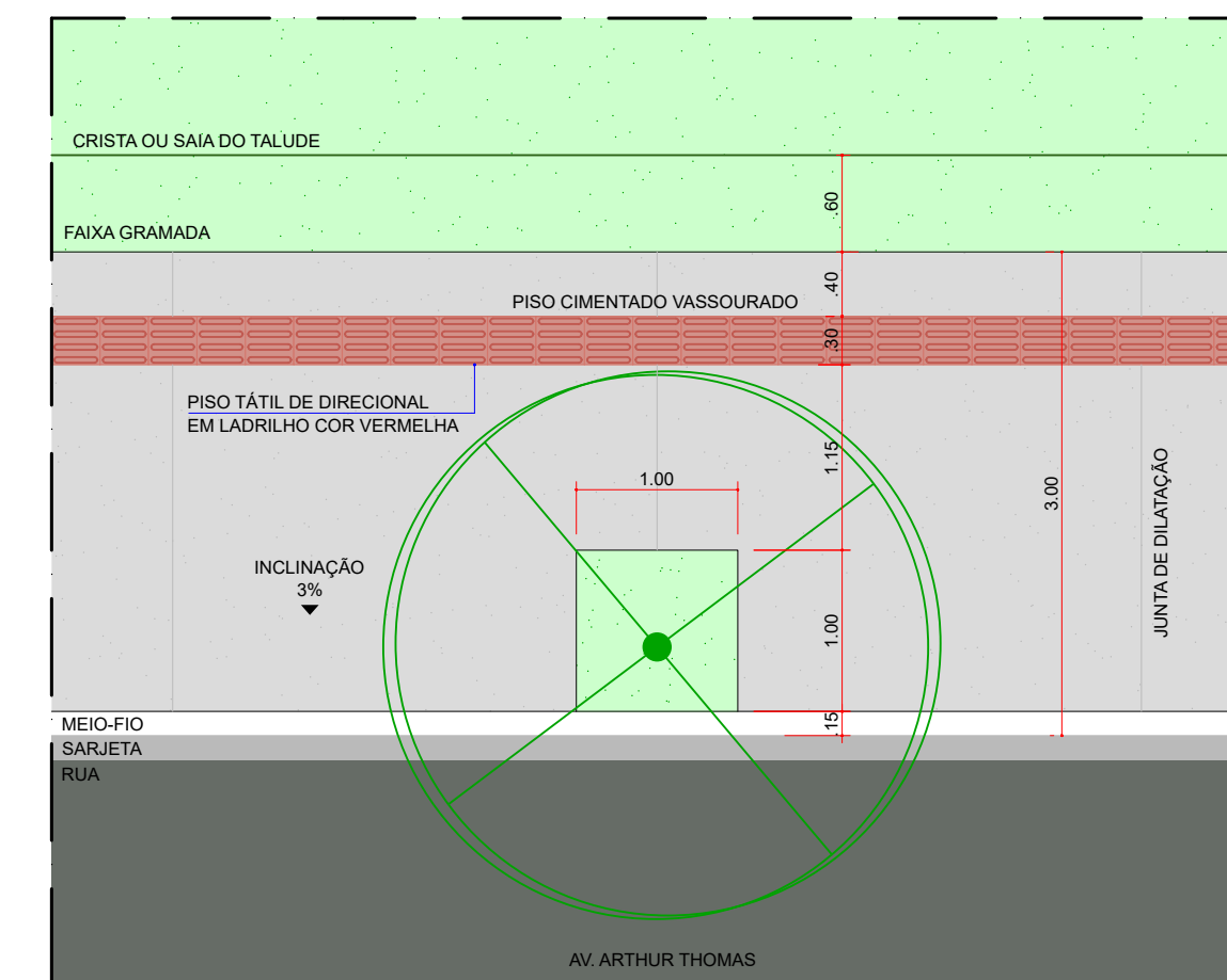
DETALHE 6 - CALÇADA COM CANTEIRO NA AV. ARTHUR THOMAS ESCALA 1:50
