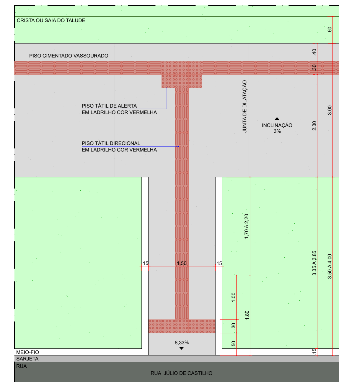
DETALHE 4 - RB2 (REBAIXO DE GUIA P.N.E. TIPO 2) ESCALA 1:50
