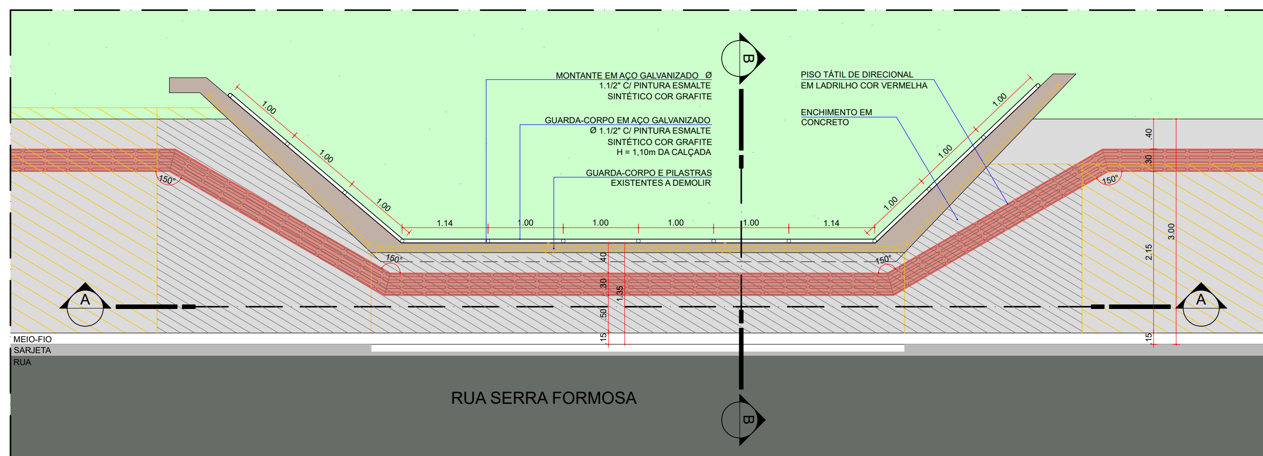
DETALHE 2 - PONTE NA RUA SERRA FORMOSA ESCALA 1:50
