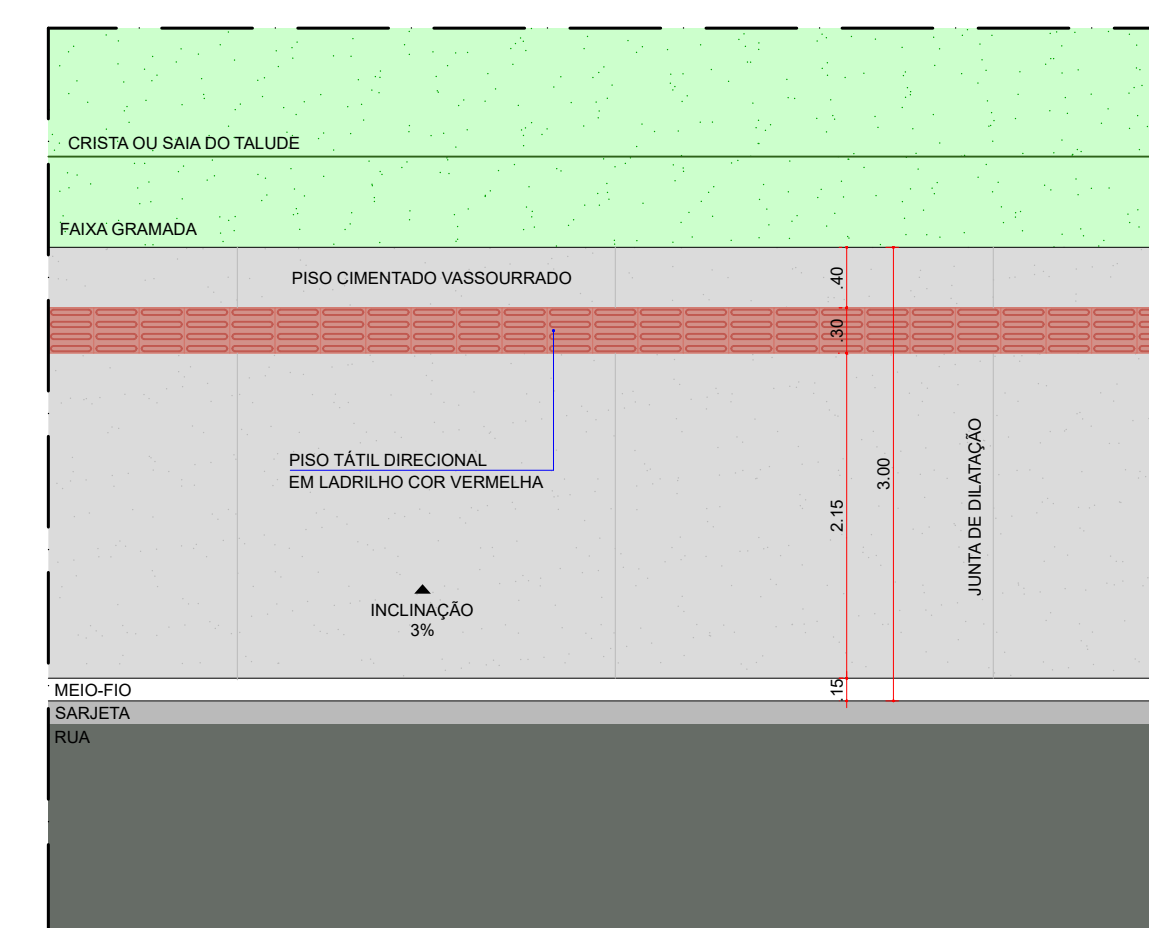
DETALHE 7 - CALÇADA SEM FAIXA GRAMADA ESCALA 1:50
