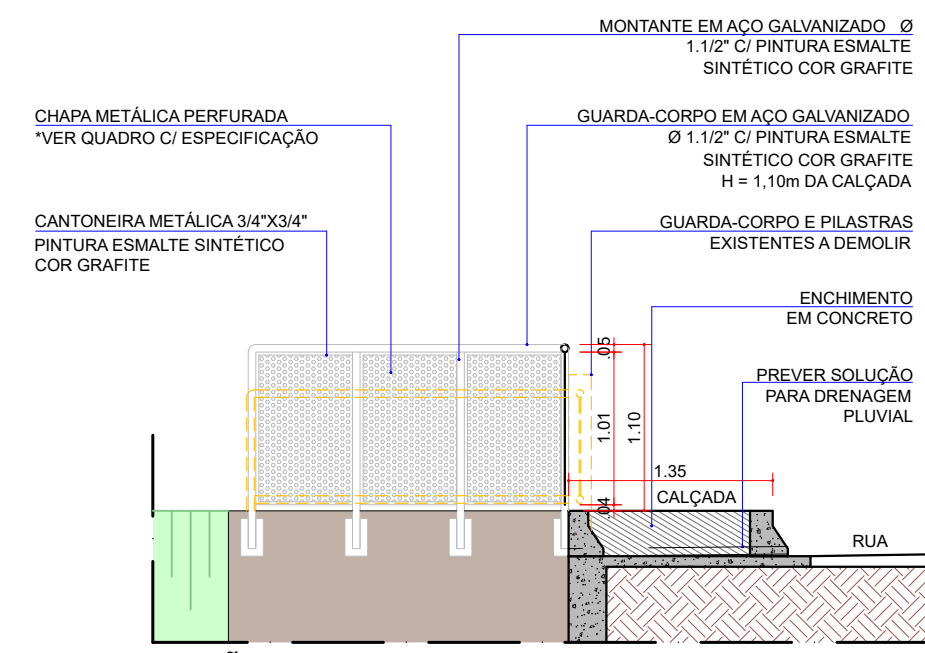
SEÇÃO BB - PONTE NA RUA SERRA FORMOSA ESCALA 1:50
