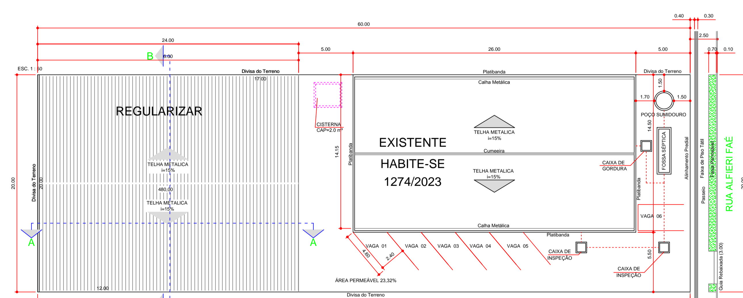
PLANTA DE LOCAÇÃO E COBERTURA ESC. 1 : 500
