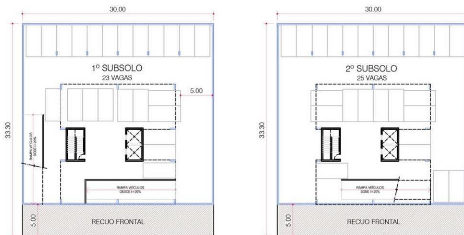
Planta Subsolos
