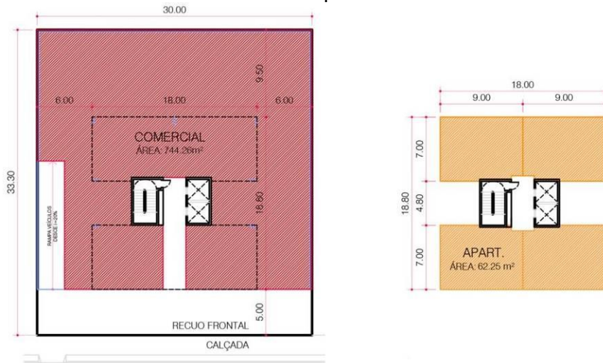
Planta Tipo
