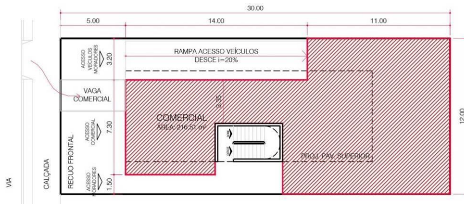
Planta Térreo
