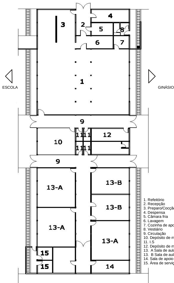
Planta Térreo – Núcleo de Alimentação e Educação Escolar Escala 1:250
