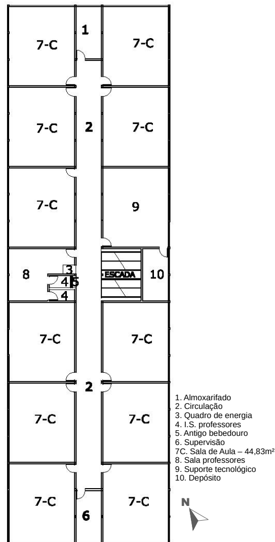
Planta Atual Superior – Bloco2 Escala 1:250
