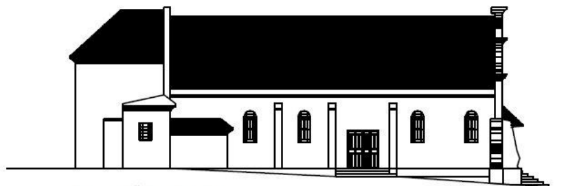
ELEVAÇÃO LATERAL
