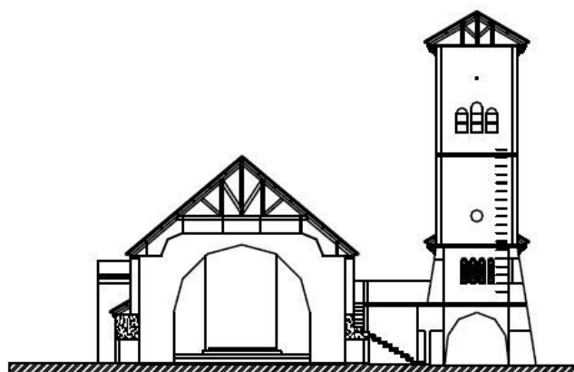
CORTE TRANSVERSAL
