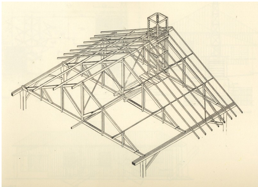
Perspectiva isométrica do madeiramento do telhado Fonte: Levantamento Antonio Carlos Zani, 1987 (ZANI, Antônio Carlos. "Arquitetura em madeira". Londrina:Eduel, 2003) Desenhos: Roberto Ikeda
