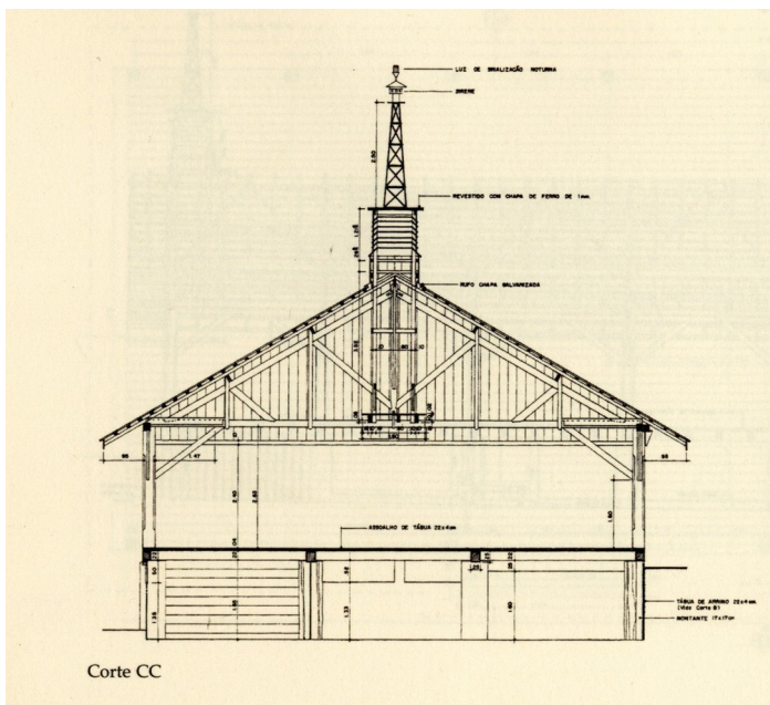
Corte Transversal
