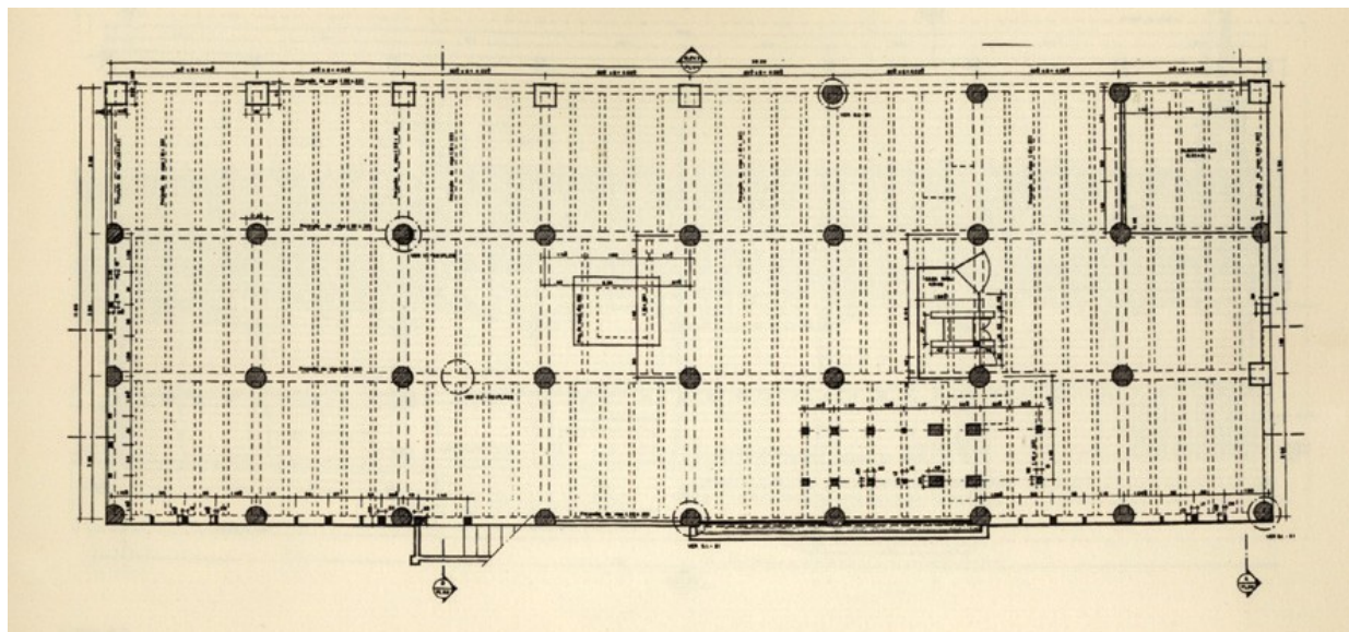
Planta do subsolo
