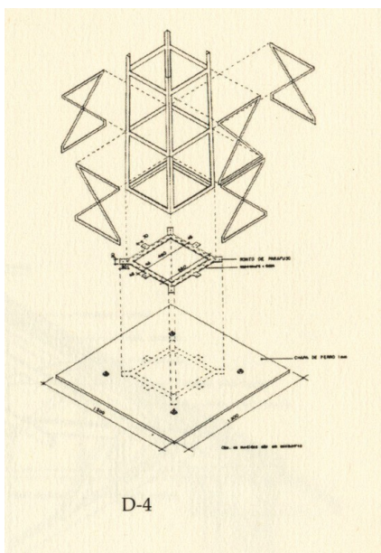
Esquema construtivo da torre Fonte: Levantamento Antonio Carlos Zani, 1987 (ZANI, Antônio Carlos. "Arquitetura em madeira". Londrina: Eduel, 2003) Desenhos: Roberto Ikeda
