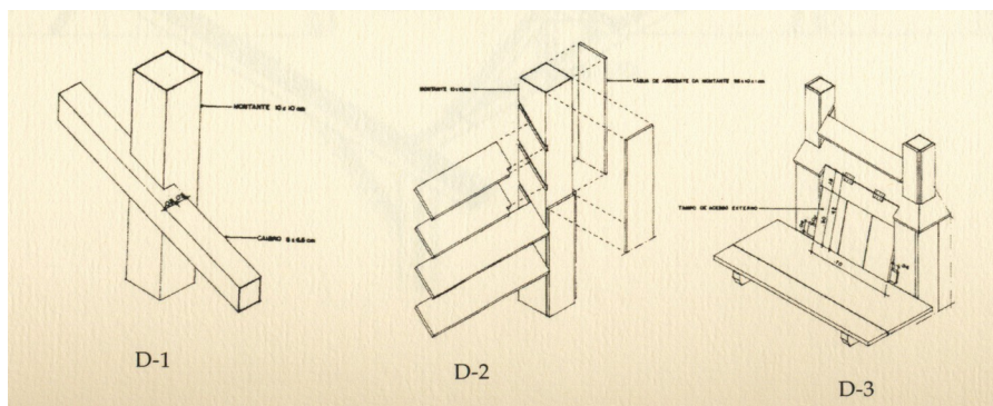
Detalhes Construtivos Fonte: Levantamento Antonio Carlos Zani, 1987 (ZANI, Antônio Carlos. "Arquitetura em madeira". Londrina: Eduel, 2003) Desenhos: Roberto Ikeda
