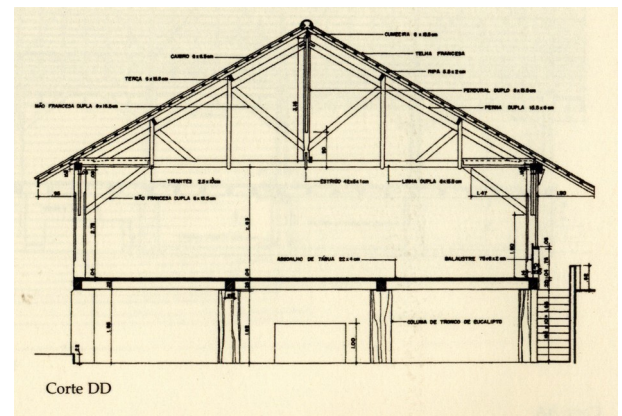
Corte Transversal
