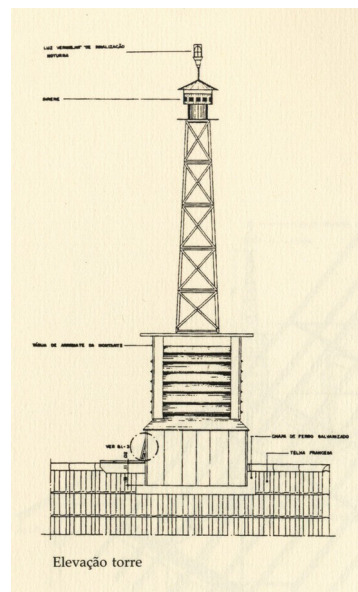
Elevação da Torre Fonte: Levantamento Antonio Carlos Zani, 1987 (ZANI, Antônio Carlos. "Arquitetura em madeira". Londrina:Eduel, 2003) Desenhos: Roberto Ikeda
