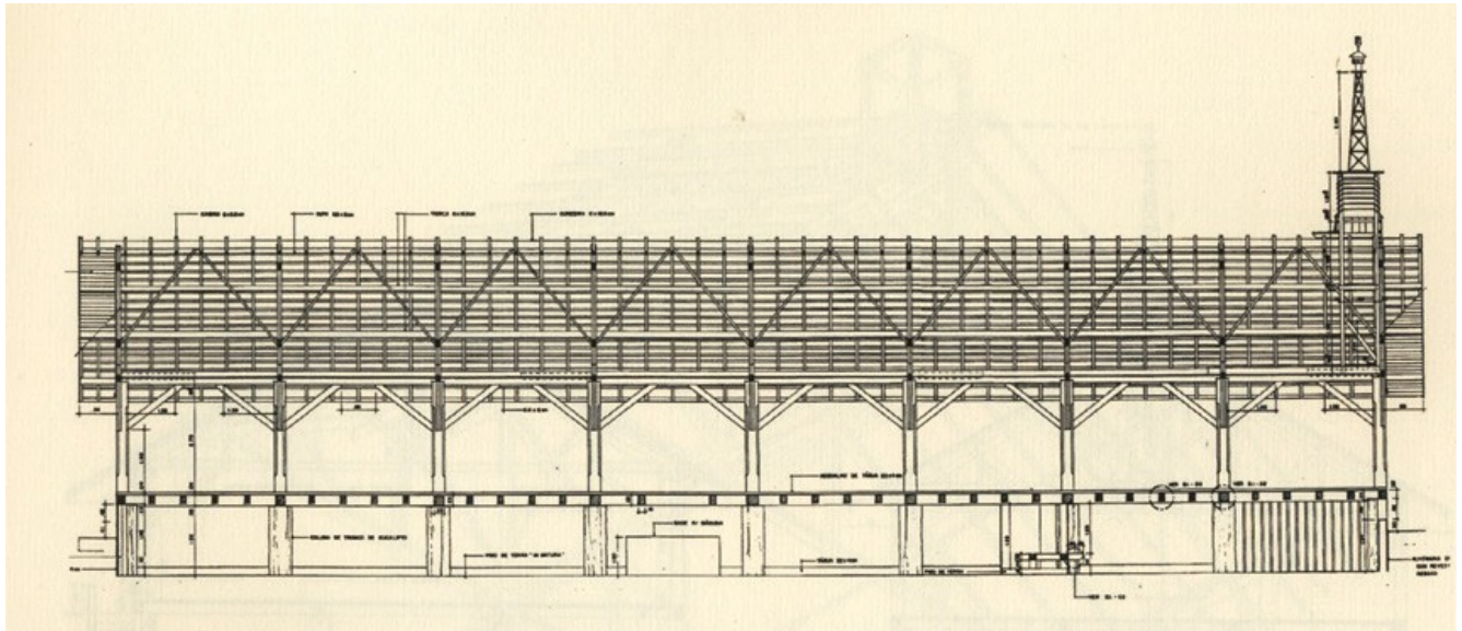
Corte Longitudinal
