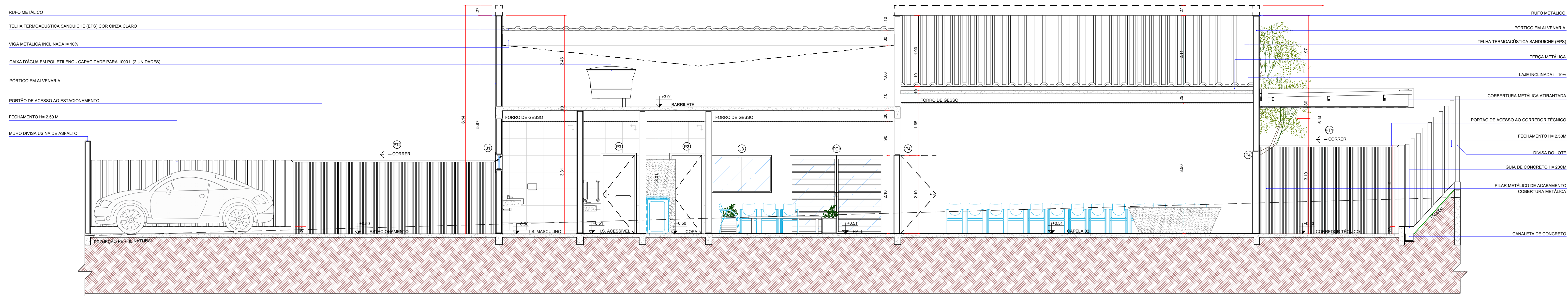
5 CORTE AA1 ESCALA 1:50
